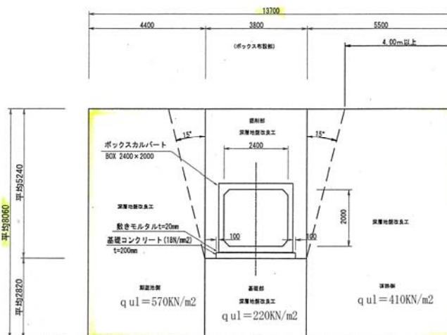
標準断面 及 改良強度
